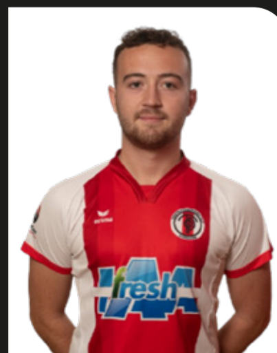
24 Lars Hüsken
